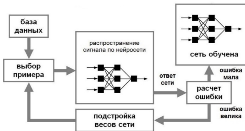
Рис. 2. Процесс обучения нейросети
