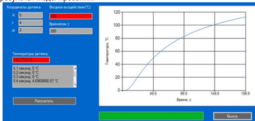
Рис. 2. Результат выполнения программы
