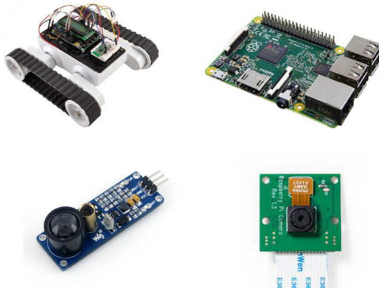
Рис. 2. Элементы системы навигации мобильным роботом на основе шасси Rover 5: Rover 5 Chassi; лазерный дальномер Камера Raspberry Pi 3
