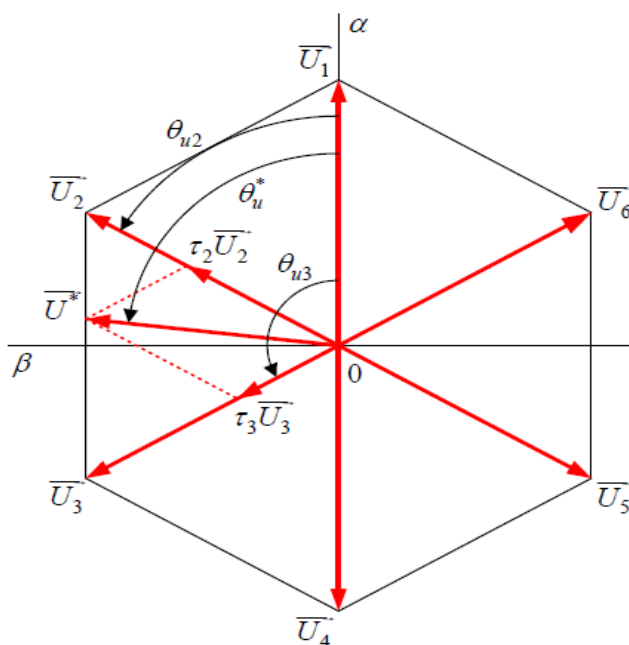
Рис. 2. Векторная диаграмма полупроводникового коммутатора
