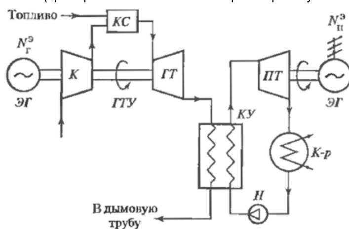
Рис. 2. Схема парогазовой установки с котлом-утилизатором
