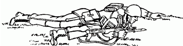
Рис. 58. Переползание по-пластунски
